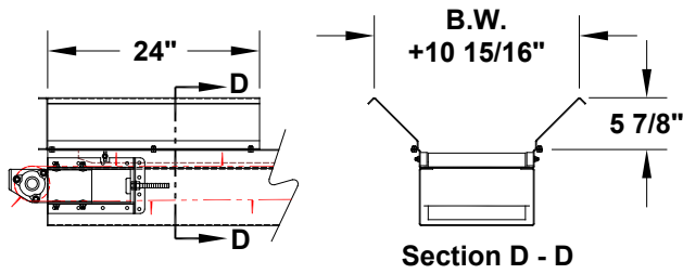
Optional Infeed Hopper
