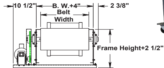
Section D-D
