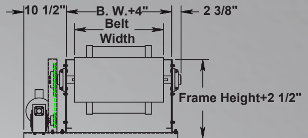
Section D-D
